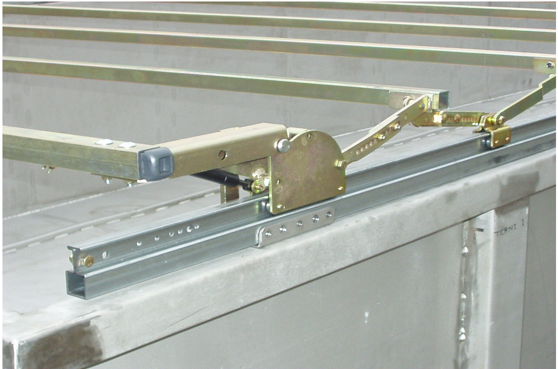
Bild 9 Verdeck - Verschluss
